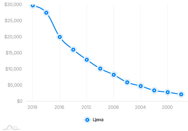
Зависимость Цена/Год
