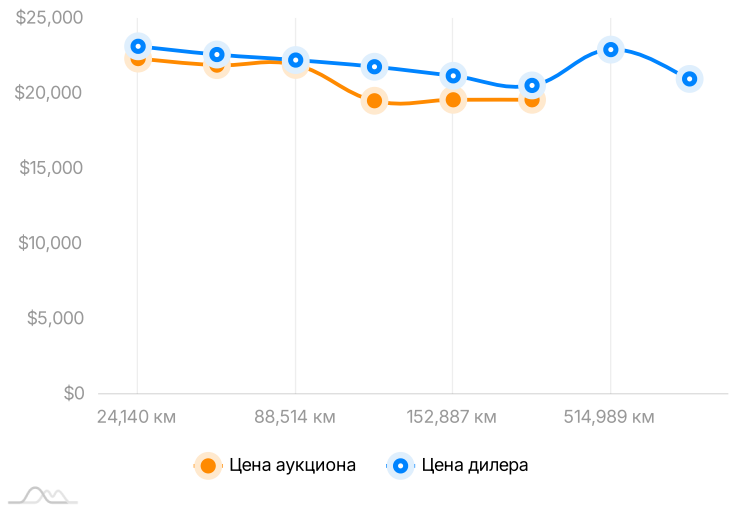
Зависимость Цена/Километраж
